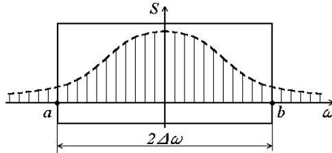
Рис. 25. К иллюстрации окна наблюдения для спектра нешумовой функции
